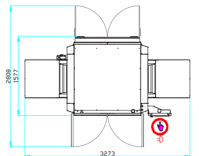
Hauteur de la machine 2384 mm
