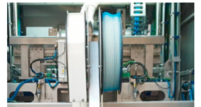
Verschlusskopf und -band wird auf Rolle bevorratet
