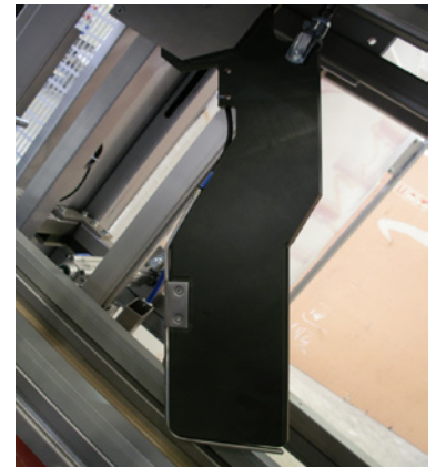
Stretcher für Kontrolle Beutelfaltung
