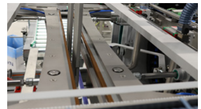
Leckdichte Beutelverschweißung
