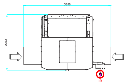
Maschinenhöhe 4870 mm
