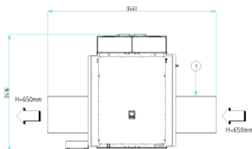
Unité de soudure à 45° en option
