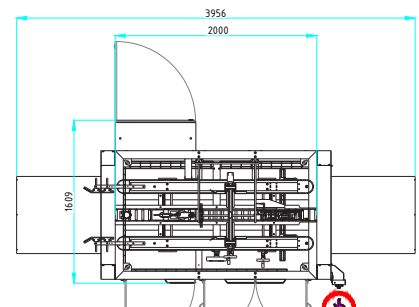
Hauteur de la machine 2385 mm
