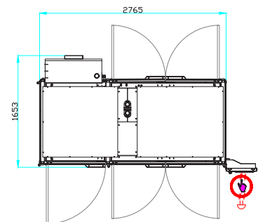
Maschinenhöhe 2133 mm
