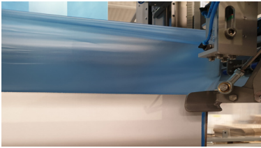
Guías para sostener las solapas
