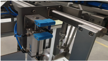
Nuevo y resistente módulo de cuchara y pinza
