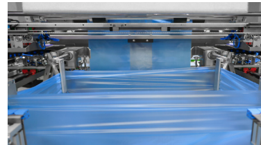
Modulo cucchiaio azionato da un servomotore
