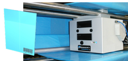
Stampante a trasferimento termico opzionale
