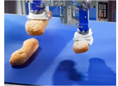
Robot con 2 ventosas individuales
