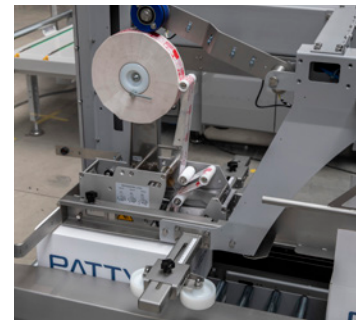
Einfache Klebebandbeladung für oberen Klebekopf
