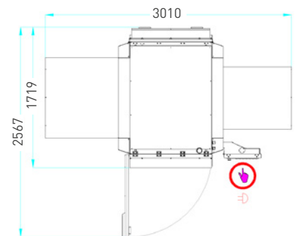
Maschinenhöhe mit Folienrollentür geschlossen: 2095 mm Maschinenhöhe mit Folienrollentür offen: 2255 mm
