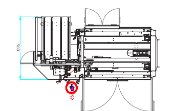
Hauteur de la machine 2384 mm
