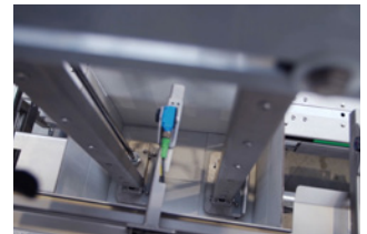
Deux plongeurs mécaniques pour un parfait collage
