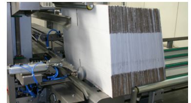
Funktionssichere Vereinzelung der Kartonzuschneite
