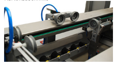
Der Karton wird an 3 Seiten gesichert
