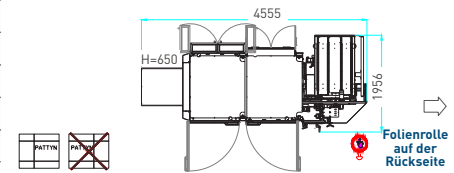
MTM 60 kg Rollen linke Heißleimversion
