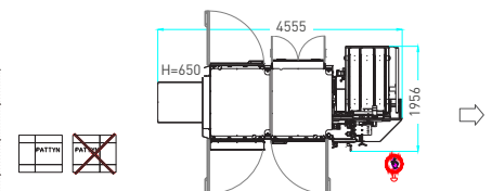
MTM/PM 12 kg Rollen linke Heißleimversion
