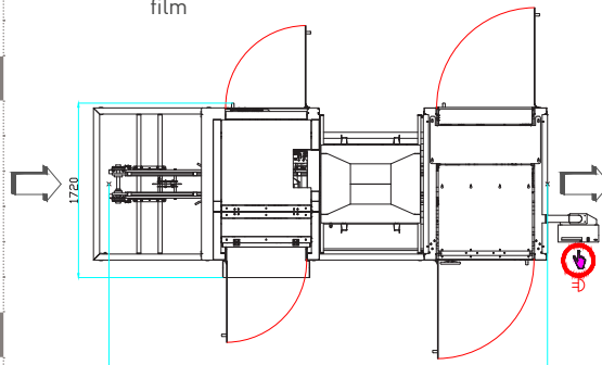
Hauteur de la machine 2126 mm
