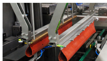
Modulo de sello superior: formación del fuelles de la bolsa y sellado
