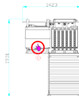
Trieuse pondérale en continu avec système d'éjection
