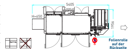
Maschinenhöhe 2090 mm
