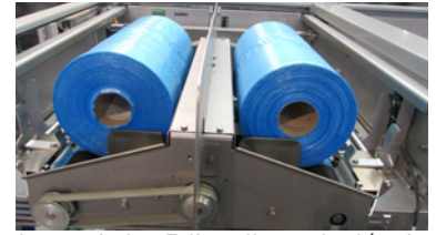
Automatischer Folienrollenwechsel (optional)
