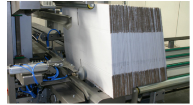
Funktionssichere Vereinzelung der Kartonzuschneide
