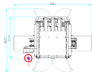
Hauteur de la machine 2621 mm
