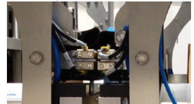
Deux doubles soudures par impulsion
