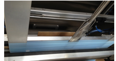
Platines d'étirement du film avec contrôle du décoiffage
