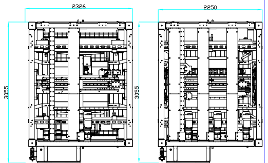
Hauteur min. de la machine 3435 mm Hauteur max. de la machine 3796 mm
