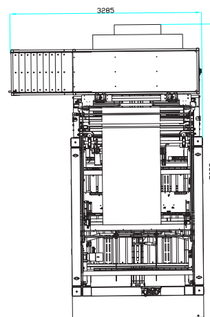
Min. hauteur de la machine 2360 mm Max. hauteur de la machine 3560 mm
