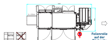
Maschinenhöhe 2090 mm
